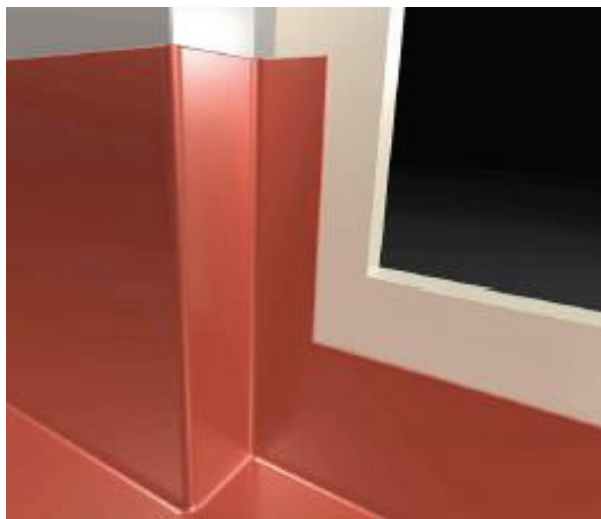
Obrázok č.4: Prechod hydroizolácie do ostenia.
